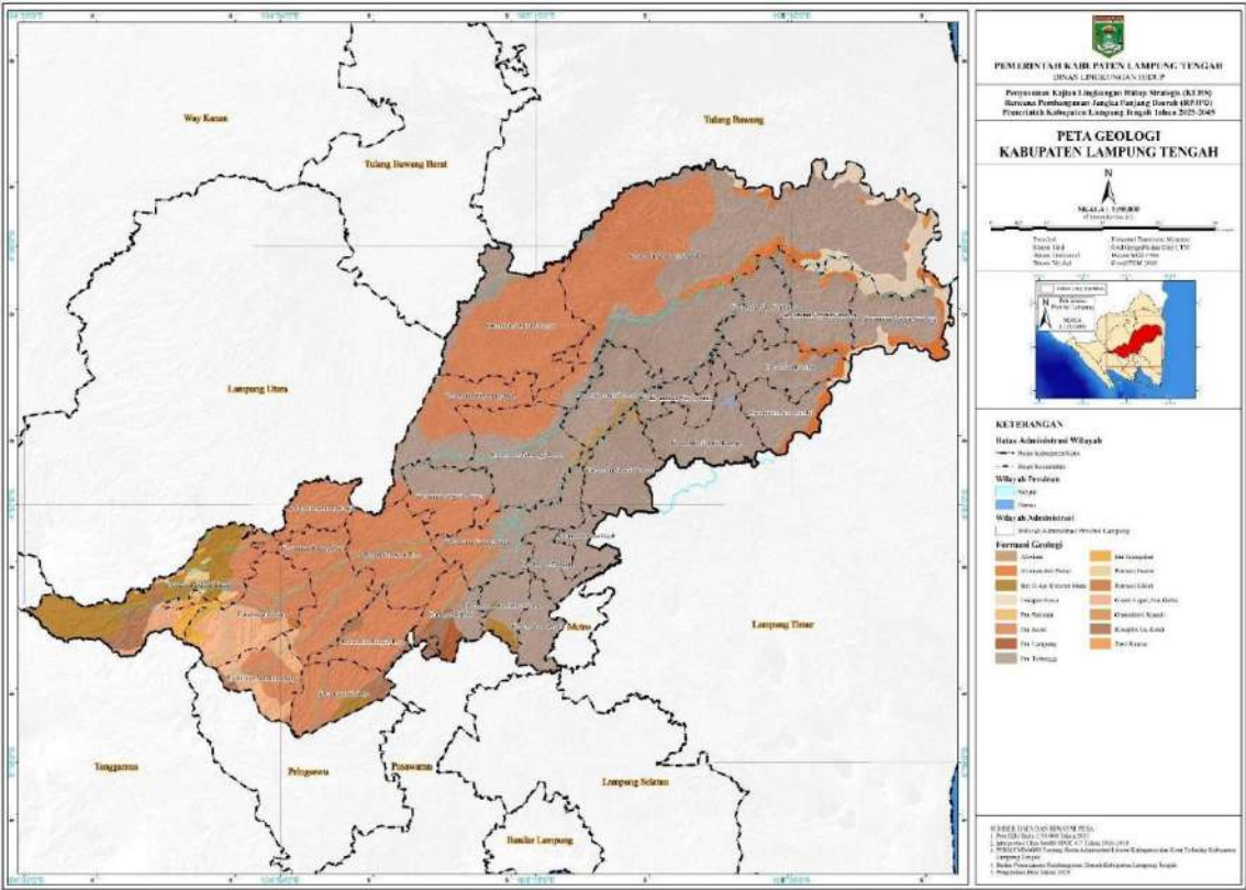
Gambar 2.4 Peta Geologi Kabupaten Lampung Tengah
