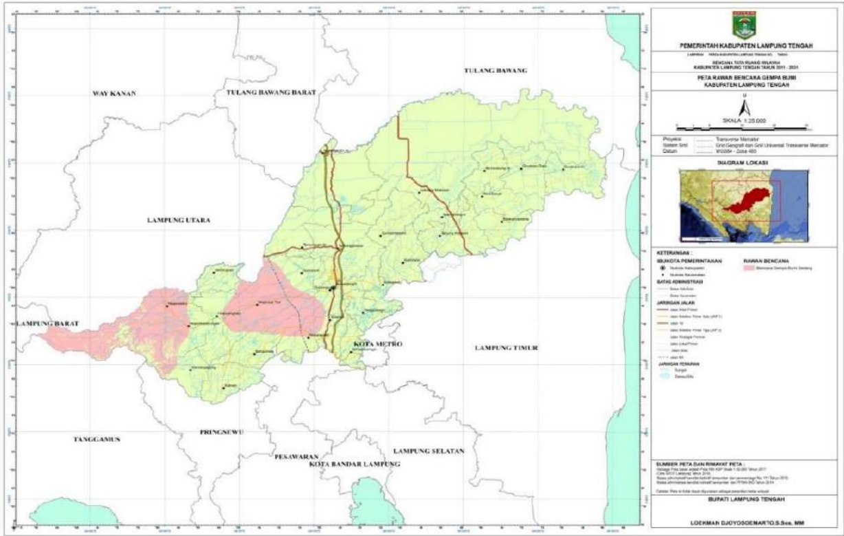
Gambar 2.11 Peta Kawasan Rawan Bencana Gempa Bumi Wilayah
